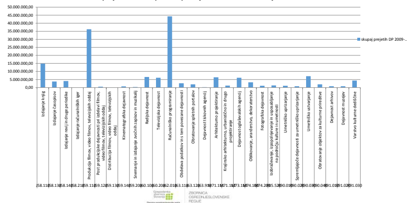
prejete državne pomoči po dejavnostih KKS v obdobju 2009-2015
