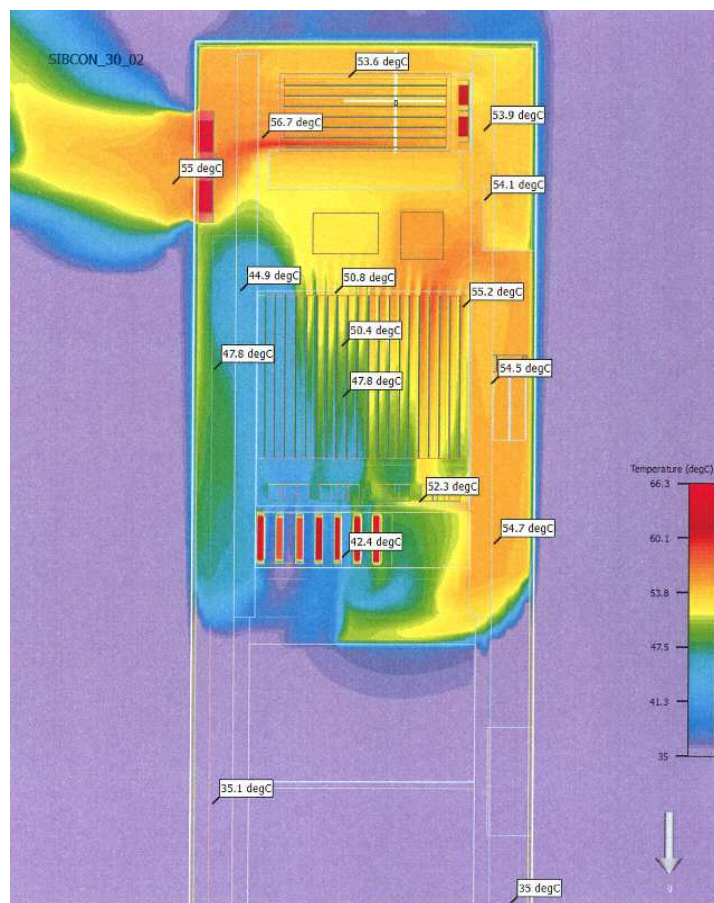
Slika 1: Temperaturne razmere pred izboljšavo ohišja SIBCON
