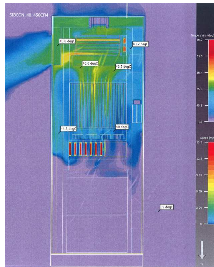
Slika 2: Temperaturne razmere po izboljšanju ohišja SIBCON
